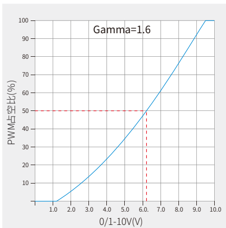
0/1-10V调光
